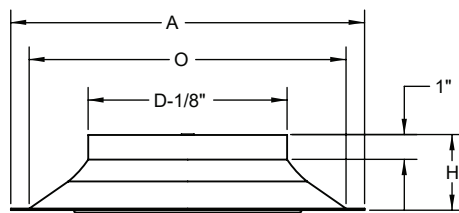
Flush Horizontal 1
